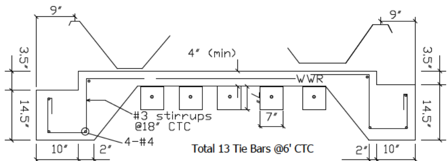
SEC A-A
